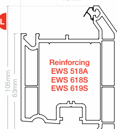
Door sash T EWS 7019
