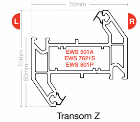
Transom Z EWS 7003
