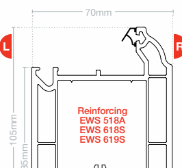
Transom Z EWS 7703
