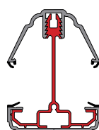
XJR1 Jack Rafter XJC25 Top Cap XBC3 Bottom Cap
