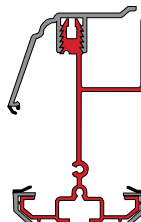
X35ER3 Wall Rafter XERC25 Top Cap XBC1 Bottom Cap
